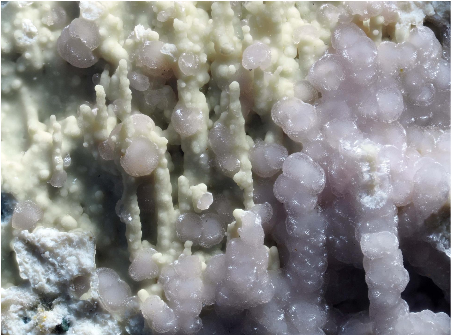
Strengite – Arbouet – Pyrénées Atlantiques champ 2,4 mm
