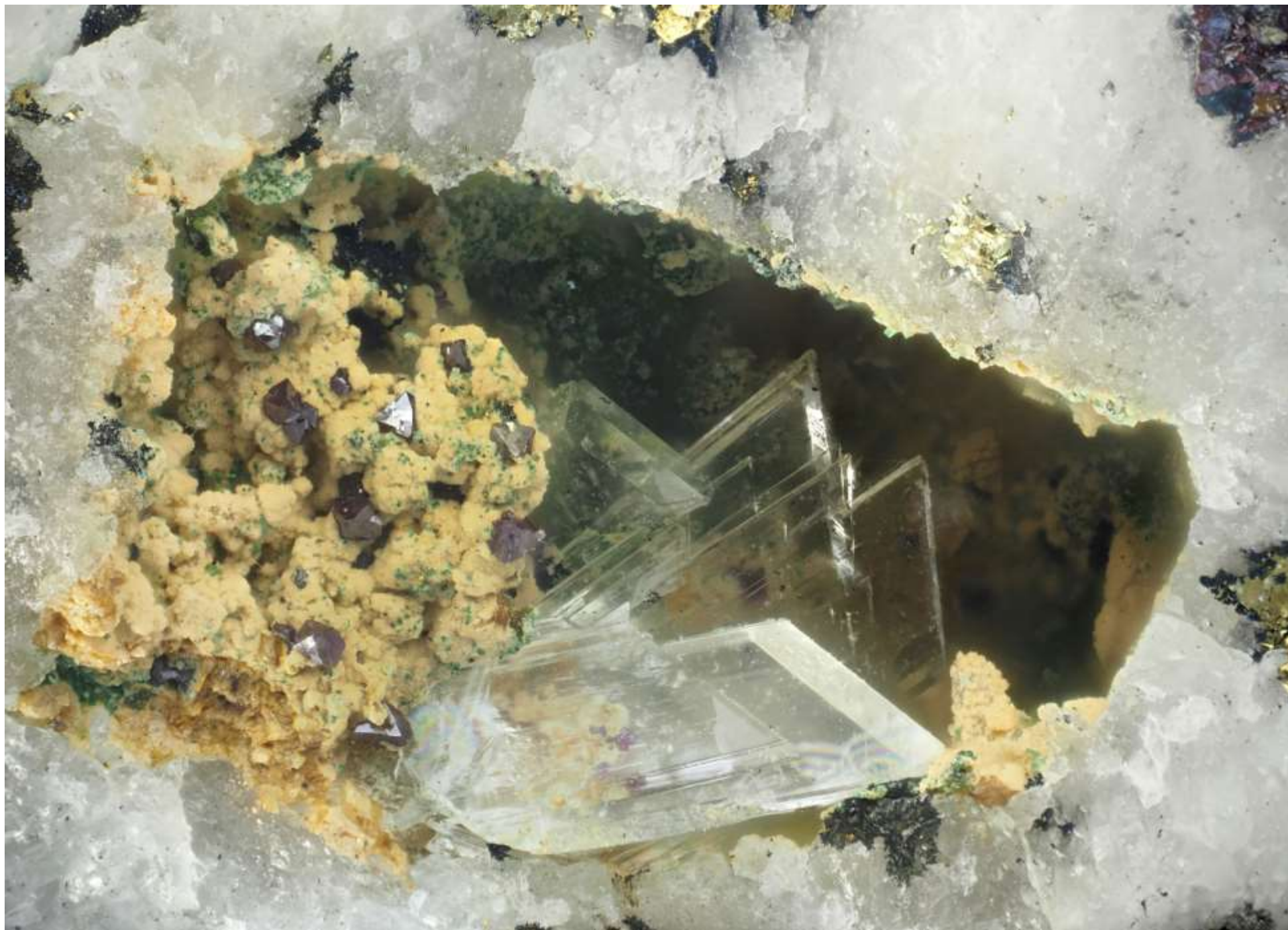
Gypse Cuprite – Papiol - Espagne champ 2,8 mm
